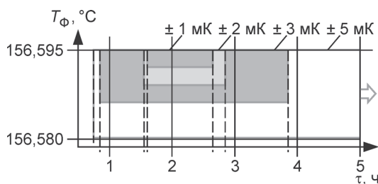
Рис. 2. Стабильность и длительность реперной точки индия при \Delta T = 0,05 К
