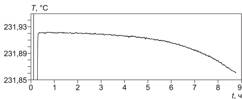
Рис. 4. Кривая затвердевания олова при температуре в калибраторе 231,80 °C
