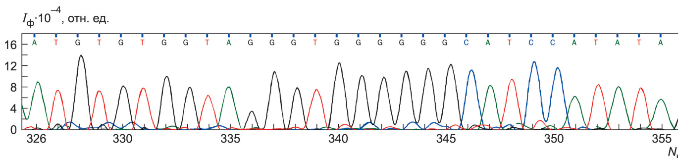
Рис. 2. Графическое изображение (электрофореграмма) последовательности фрагмента ДНК, полученное на генетическом анализаторе Нанопор 05; I_\phi – интенсивность флуоресценции; N_n – порядковый номер нуклеотида; буквы – нуклеотиды, пики – сигнал флуоресценции
