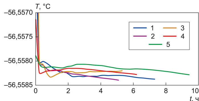
Рис. 2. Воспроизводимость значения температуры тройной точки \text{CO}_2 с использованием ампулы 1 при четырех независимо замороженных мантиях (кривые 1–4) и ампулы 2 (кривая 5)
