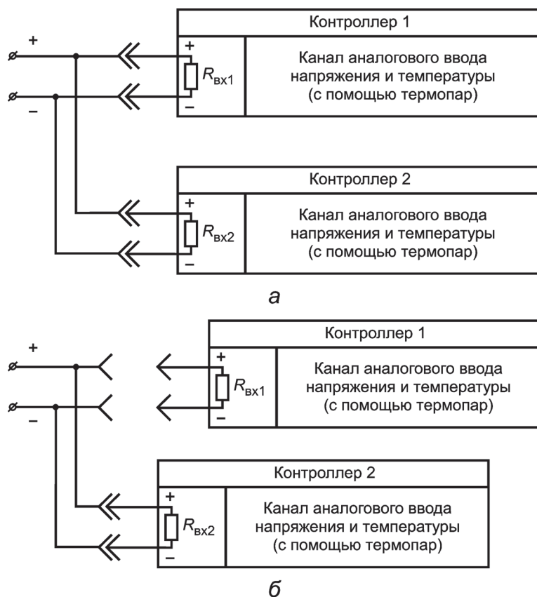
Рис. 3. Схемы резервирования канала ввода напряжения термопреобразователя: рабочее состояние основного и резервного каналов измерений (а) и режим замены основного канала измерений (б)
