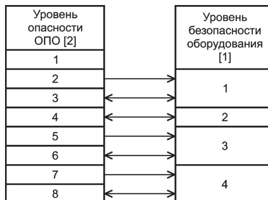
Рис. 1. Схема соответствия уровней опасности ОПО уровню безопасности оборудования
