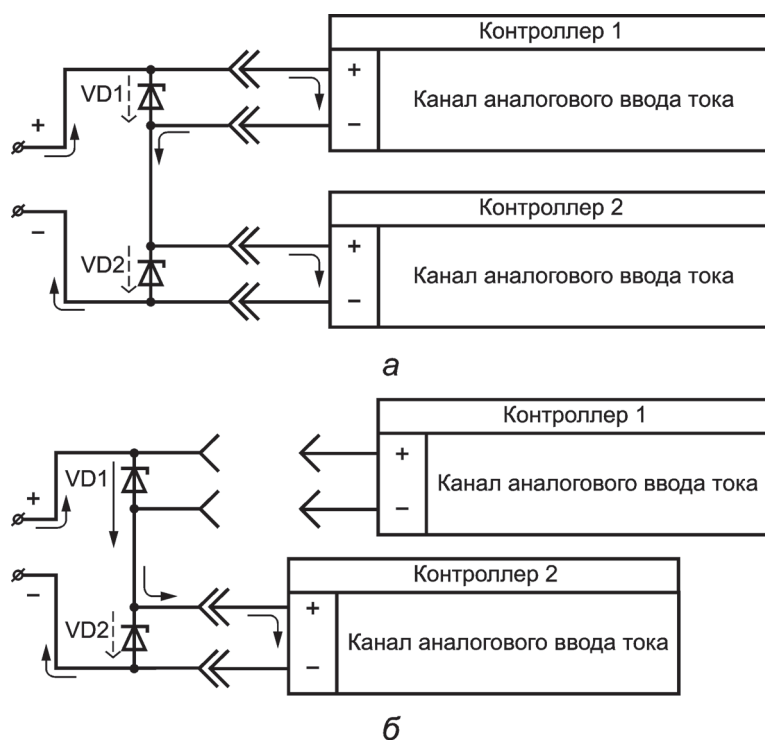
Рис. 2. Схемы резервирования канала токового ввода: рабочее состояние основного и резервного каналов измерений (а) и режим замены основного канала измерений (б); VD1, VD2 — стабилизаторы
